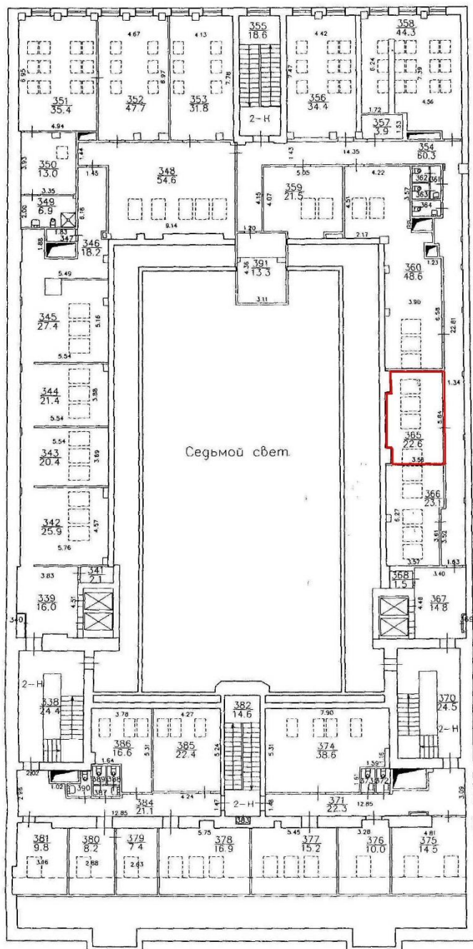
План мансарды
